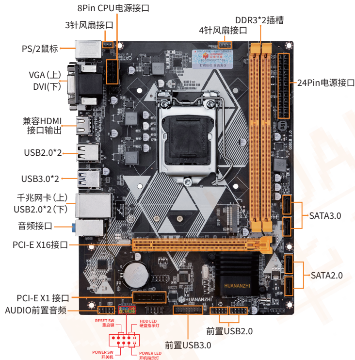
图1-1 B85主板图解
